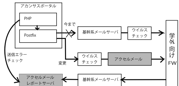
図 16 アクセルメール導入のシステム構成
